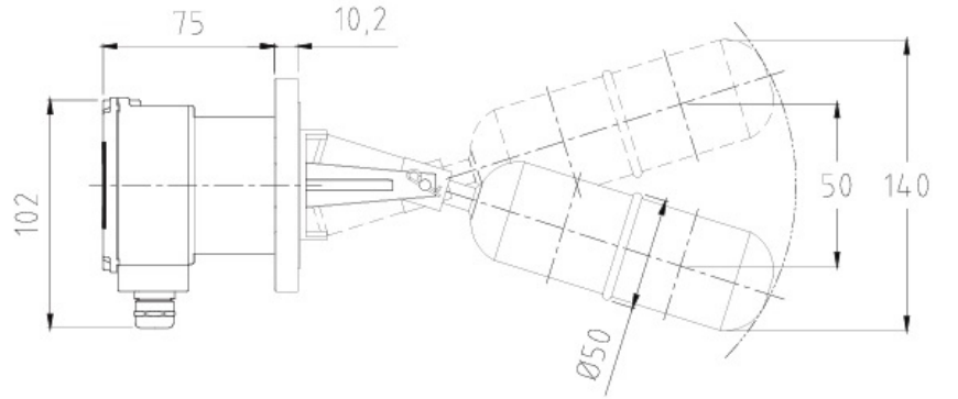
F SEVİYE ŞALTERİ ÖLÇÜLERİDİR.
