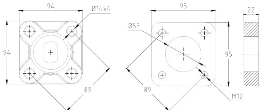
F SEVİYE ŞALTERİ ÖLÇÜLERİDİR.
