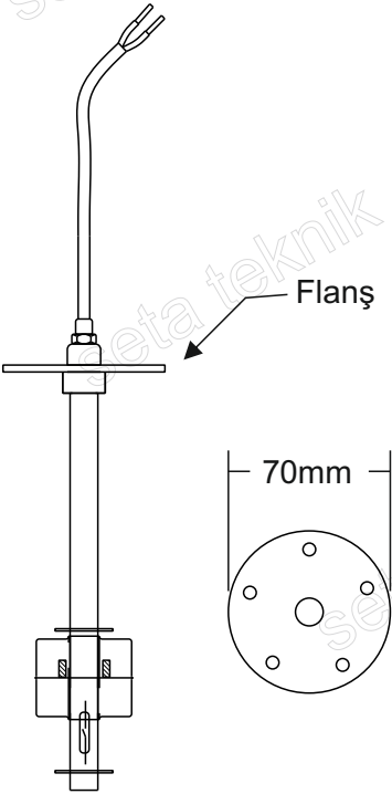
Flanşlı Montaj Aparatı Ø70mm
