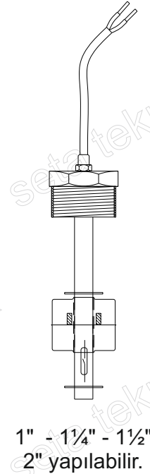
Dış Dişli Montaj Aparatı
